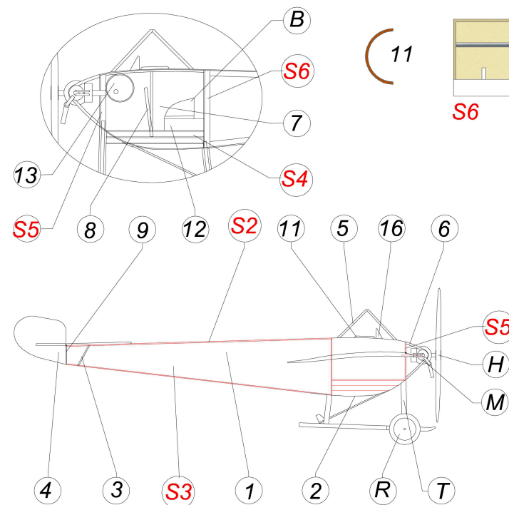
H hélice CHAUVIERE rotation horaire vue place pilote
